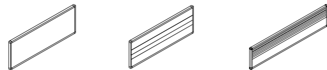
Fabric/Tackable/Acoustic/White Steel Panel 布屏风 / 针板屏风 / 吸音 / 金属白板 W: 900,1100,1200,1300,1400, 1500,1600,1700,1800 H: 356,462
