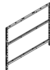
Metal Frame 金属框架 W: 400-1800 H: 1100,1207,1507,1657,1807
