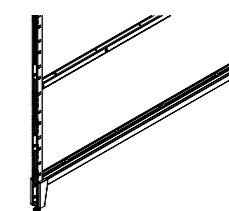
High Foot Panel 高脚 W: 400-1800 H: 150
