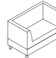
1100 Armed Sofa/1100 带扶手沙发 w/Fixed Panel/Drawer 带底格固定面板 / 抽屉 W1100 D595 H745 W1100 D695 H745
