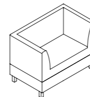
1000 Armed Sofa/1000 带扶手沙发 w/Fixed Panel/Drawer 带底格固定面板 / 抽屉 W1000 D595 H745 W1000 D695 H745
