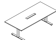
Rectangular Desk 直会议台 W : 2000,2200 H : 800,900,1000
