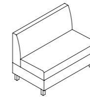
900 Armless Sofa/900 无扶手沙发 w/Fixed Panel/Drawer 带底格固定面板 / 抽屉 W900 D595 H745 W900 D695 H745
