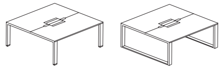
Double-sided Bench for 2 Person 对座台 · 2 人 W: 1200, 1400, 1500, 1600 D: 1200, 1400 H: 745
