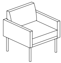
1-Seater Sofa, Half Height Arm 一人位沙发·半高扶手 W700 x D700 x H745
