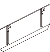
Metal Modesty Panel Hanging on Bar 金属前挡板·横杆悬挂 W: 900, 1100, 1200, 1300 T: 12 H: 320
