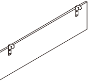
MFC Modesty Panel Fixed on Top 三聚氰胺板前挡板·台底固定 W: 900, 1140, 1240, 1340 T: 16 H: 350
