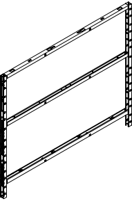
Metal Frame 金属框架 W: 400-1800 H: 1100,1207,1507,1657,1807
