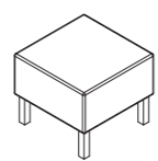
Mini Ottoman w/ Metal Leg 脚垫，金属脚 DNOM() - W460 x D460 x H420
