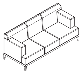
Sofa, 3 seat 三位沙发 MYS-3S ( ) - W2100 x D850 x H880
