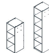
Bookcase 组合柜书架 H : 1205, 1353, 1950, D : 400, 470 W : 450
