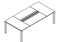
Conference Table 会议桌 H : 745 D : 1200, 1400, 1600 W : 1400, 2400, 3000, 3500, 4000
