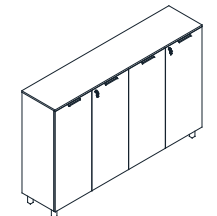
Middle cabinet w/ 4 swing doors 中柜·带四掩门 H : 1370 D : 470 W : 2080
