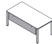
Modesty panel 前挡板 H : 400 W : 1270, 1470, 1670
