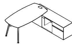
MAIN DESK W/SIDE CABINET 主桌带边柜 W1800 D1310 H748 W2000 D1340 H748 W2200 D1340 H748 W2380 D1350 H748
