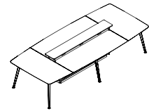
CONFERENCE TABLE W/O TOWER 会议桌带盒子 W2800 D1500 H891 W3400 D1500 H891 W4000 D1500 H891
