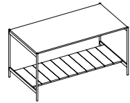
Social Table 社交高桌 W: 1630, 2030 D: 1090 H: 1050
