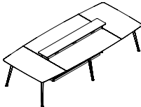
CONFERENCE TABLE W/O TOWER 会议桌上盒子 W2800 D1500 H891 W3400 D1500 H891 W4000 D1500 H891
