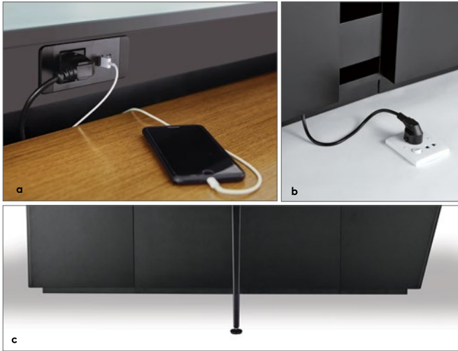
a CONVENIENT POWER AND USB SOCKET SUPPORTS BYOD b SLIDING DOOR OPENING FOR THE EASE OF CABLE MANAGEMENT c MODULAR DESIGN TOWER BASE ALLOWS ITS' 600MM SEGMENTS TO EXTEND THE TABLE UP TO 9.8M a 便捷的电源和USB插座可连接自携装置 BYOD，能提供即插即用功能 b 底座趟门设计，方便走线管理 c 底座模组化设计，可不断增加600毫米底座模组，使会议桌最长伸展至9.8米
