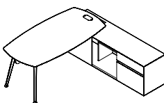
MAIN DESK W/EXTENDED CABINET 主桌带长边柜 W1800 D1910 H748 W2000 D1940 H748 W2000 D2330 H748 W2200 D1940 H748 W2200 D2330 H748 W2380 D1950 H748 W2400 D2350 H748
