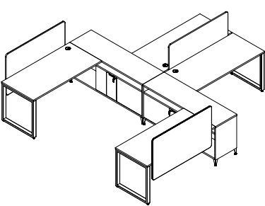
Cluster of 4 workstations, Dual Cabinet w/Open Shelf & Swing Door 四人工位 双边矮柜，带掩门，空格柜
