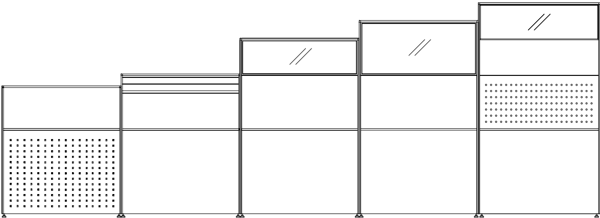
Top : Painted Flat Metal Bottom : Perforated Metal, Embossed Metal 顶板 : 平板金属 底格 : 方孔金属， 美案板金属
