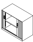
Fixed Metal Roller Shutter Door Cabinet 钢制固定卷门边柜 W: 800-1200 D: 450,470 H: 710,900
