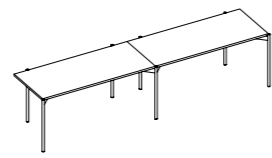
Single Bench 单边共享台 W: 1230, 1430, 1530, 1630 D: 660, 760, 810 H: 740
