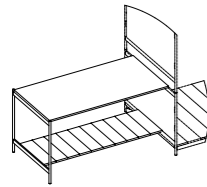
Social Table 社交高桌 W: 1630, 2030 D: 1090 H: 1050
