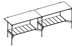
Single High Bench 单边站立共享台 W: 1230, 1430, 1530, 1630 D: 660, 760, 810 H: 1050
