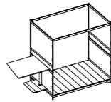
Pavilion* (Without Curtain) 多功能舱* (不包括窗帘) W: 2230 D: 1290, 1490, 1590 H: 2300
