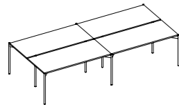
Bench 共享台 W: 1230, 1430, 1530, 1630 D: 1290, 1490, 1590 H: 740
