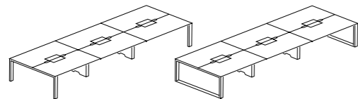
Double-sided Bench for 6 staffs 对座台 · 6 人 W: 3600, 4200, 4500, 4800 D: 1200, 1400 H: 745
