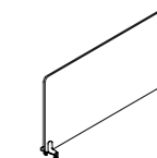
Frameless Fixed Screen 无框扞布固定屏风 W: 1395, 1495, 1595 H: 750 T: 20
