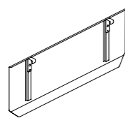
Metal Modesty Panel Hanging on Bar 金属前挡板·横杆悬挂 W: 900, 1100, 1200, 1300 T: 12 H: 320
