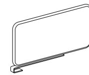
Desktop Divider Screen 分隔桌上屏风 W: 600, 700, 800 D: 25 H: 356
