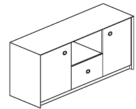
Low CAB w/ 2 SW & DR& Open shelf 矮柜带两个掩门, 抽屉, 空格 W1200 x D400 x H796
