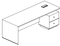
Main desk w/ Pedestal, CN/HK socket, wood leg 主桌带柜桶, 中式 / 英式插座 可选, 木脚 W1800 x D900 x H760 W2000 x D900 x H760
