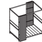
Pavilion*2 (With Slatted Screen) 多功能舱*2 (包括木条屏风) W: 2230 D: 1290, 1490, 1590 H: 2300
