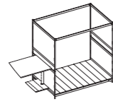
Pavilion*1 (Without Curtain) 多功能舱*1 (不包括窗帘) W: 2230 D: 1290, 1490, 1590 H: 2300
