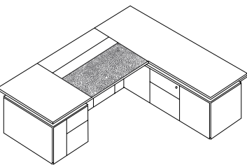
Executive Desk, w/Extended Drawer Cabinet 行政主桌带长边柜连抽屉 W3800 D2800 H760 W3600 D2800 H760 W3400 D2600 H760 W3200 D2600 H760 W3000 D2400 H760 W2800 D2400 H760 W2400 D2200 H760
