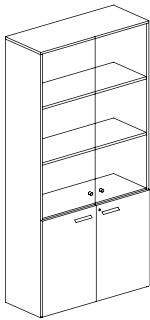
High Cabinet w/Glass and Wood Door 4 门高柜（上玻璃，下木门） W800 D420 H2000 W1000 D420 H2000
