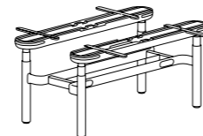
HAB Adjustable Leg 共享升降脚架 W: 1400,1500,1600,1800 H: 600, 700
