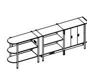
Open Shelf 3 Tiers w/ Locker 三层置物架配储物柜 W3320 D560 H1050
