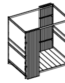
Pavilion (with Slatted Screen) 多功能舱 (包括木条屏风) W2200 D1485 H2300 W2200 D1685 H2300 W2200 D1785 H2300
