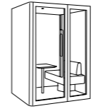
1-2P Lounge 1-2 人休闲间 W1600 D1300 H2200
