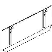
Metal Modesty Panel Hanging on Bar 金属前挡板·横杆悬挂 W: 940, 1100, 1200, 1300 T: 12 H: 320
