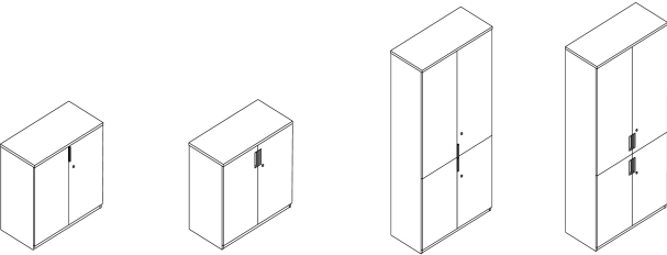
W700/800/900/1000/1100/1200 D400/450 H745/900/1145/1300/1700/2100 (L Shape/Embedded Handle) (可选 L 型 / 内嵌拉手)
