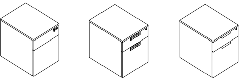
Pedestal 2 Drawers W427 D555 H523 (L Shape/Embedded/Slope Edge Handle) 2 斗可坐抽屉柜 (L 型 / 内嵌 / 斜边拉手)
