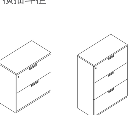
W800/900/1000 D450 H745/1145 (L Shape/Embedded Handle) (可选 L 型 / 内嵌拉手)
