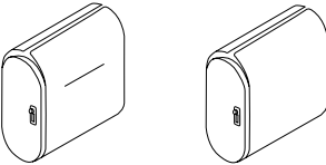
Pocket (L/R) 台底悬挂式储物柜 (左 / 右) W: 220 D : 440 H : 500
