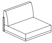
1-Seater Sofa, Armless 一人位沙发·无扶手 W700 x D700 x H465
