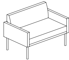
2-Seater Sofa, Half Height Arm 两人位沙发·半高扶手 W1100 x D1100 x H745 W1400 x D1100 x H745 W1500 x D1100 x H745 W1600 x D1100 x H745
