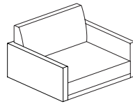
1-Seater Sofa, Two Arms 一人位沙发·两扶手 W700 x D700 x H465
