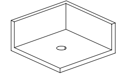
Corner Table for Wireless Charger 转角茶几用于安装无线充电器 W690 x D690 x H310
