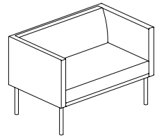
2-Seater Sofa, Full Height Arm 两人位沙发·高扶手 W1100 x D1100 x H745 W1400 x D1100 x H745 W1500 x D1100 x H745 W1600 x D1100 x H745
