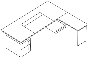
Executive Desk w/pedestal, return cabinet 主桌·连抽屉柜及边柜 W1800 D1880 H750 W2000 D1880 H750 W2200 D2000 H750 W2400 D2000 H750
