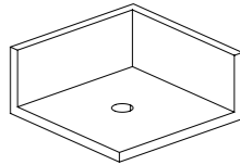
Corner Table for Wireless Charger 转角茶几用于安装无线充电器 W690 x D690 x H310
