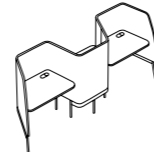
Triple Workpod 三人工作站 W2785 D730 H1300 W2785 D730 H1500
