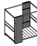
Pavilion (with Slatted Screen) W2200 D1485 H2300 W2200 D1685 H2300 W2200 D1785 H2300
