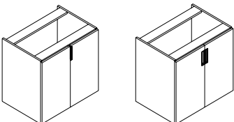
(L Shape/Embedded Handle ) (可选 L 型 / 内嵌拉手) W766 D540 H720
