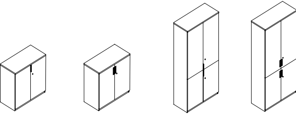
(L Shape/Embedded Handle ) (可选 L 型 / 内嵌拉手) W700/800/900/1000/1100/1200 D400/450 H745/900/1145/1300/1700/2100
