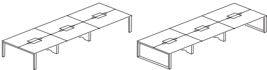
Double-sided Bench for 6 staffs 对座台 · 6 人 W: 3600, 4200, 4500, 4800 D: 1200, 1400 H: 745
