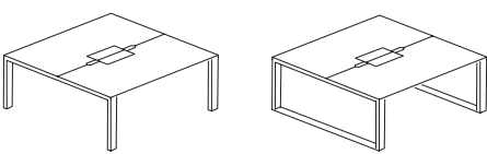
Double-sided Bench for 2 staffs 对座台 · 2 人 W: 1200, 1400, 1500, 1600 D: 1200, 1400 H: 745
