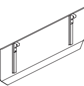
Metal Modesty Panel Hanging on Bar 金属前挡板·横杆悬挂 W: 940, 1140, 1200, 1300 T: 12 H: 320
