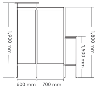
Double Touchdown 双边临时工作亭 Top View 俯视图 / Elevation 立面图
