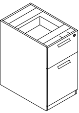
Fix Pedestal (2 drawers) 两抽固定柜 W: 380 D: 600, 700 H: 720
