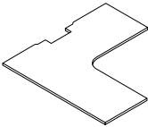
L-Shaped Desk Top L 形台面 W1：1400,1500,1600 D1：600,700 W2: 1200,1400,1500,1600 D2：600,700
