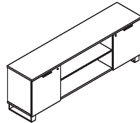
Low cabinet 矮柜 H : 732 D : 470 W : 2080
