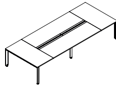
Conference Table 会议桌 H : 745 D : 1200, 1400, 1600 W : 2400, 2800, 3000, 3200, 3500, 4000
