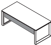
Modesty panel 前挡板 H : 400 W : 760 - 1410
