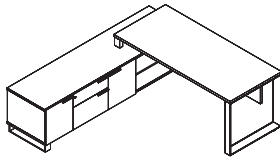
Main desk w/ credenza 主桌带边柜 Main desk 主台 H : 745 D : 800, 900 W : 1600, 1800, 2000 Credenza 边柜 H : 745 D : 600 W : 1800, 2200
