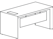
Main Desk 主桌 W: 1600 W: 1800 W: 2000 D: 800 D: 900 D: 900 H: 760 H: 760 H: 760
