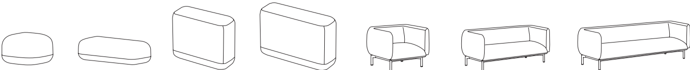
Pouf 座墩 W620 D620 H430 Cushion 座垫 2-Seater 双座位： W1200 D620 H430 3-Seater 三座位： W1360 D620 H430 Armrest 扶手 W950 D350 H660 Backrest 靠背 2-Seater 双座位： W1200 D350 H660 3-Seater 三座位： W1360 D350 H660
