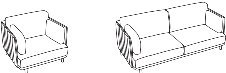
1-Seater Sofa 单座位沙发 W980 D840 H800 3-Seater Sofa 三座位沙发 W1820 D840 H800
