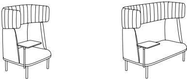
1-Seater Sofa, w/ or w/o Tablet 单座位卡座沙发，不带或带 书写板 W930 D760 H1260 2-Seater Sofa, w/ or w/o Tablet 双座位卡座沙发，不带或带 书写板板 W1540 D760 H1260
