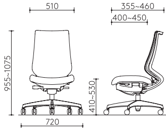
High Back Chair without Armrest 高背座椅不带扶手
