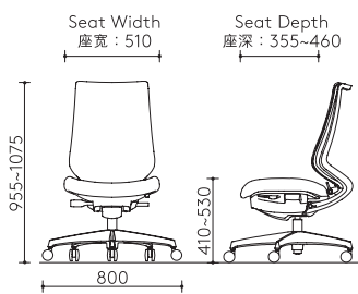
High Back Chair without Armrest 高背座椅不带扶手
