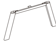
A-Shape Leg A形脚 Single Bench 单边共享台 W: 600, 700, 750 H: 725 Double Bench 双边共享台 W: 1200, 1400, 1500 H: 725
