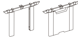
Straight Leg w/ or w/o Cable Cover 直形脚 带/不带 走线盖 Single Bench 单边共享台 W: 600, 700, 750 H: 725 Double Bench 双边共享台 W: 1200, 1400, 1500 H: 725
